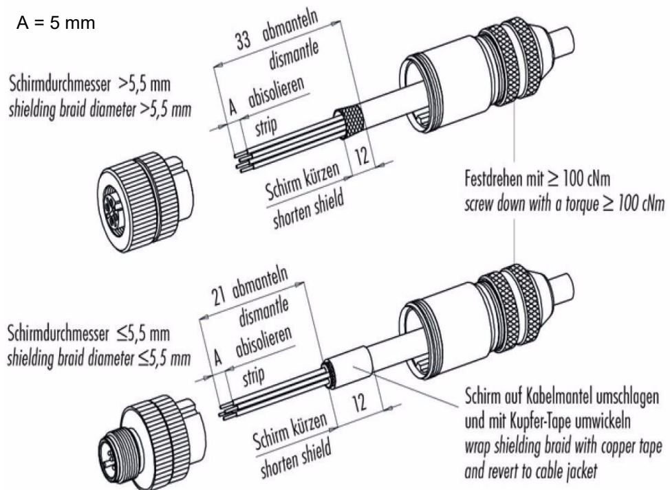
Fig. 55: Connecteur M12, à 5 pôles pour l'interface analogique
