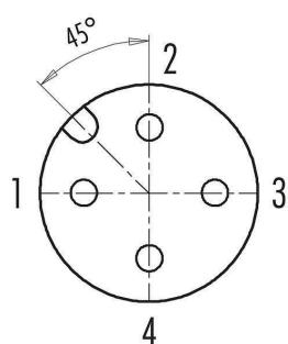
Fig. 10: Affectation des broches de l'entrée de capteur
